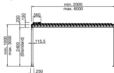
Zijaanzicht
